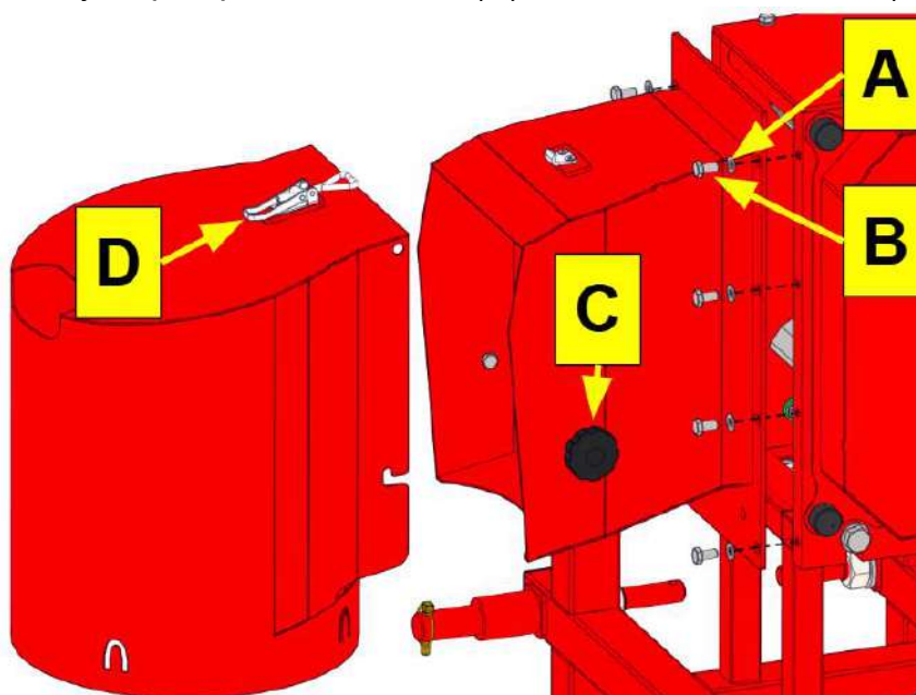
Рисунок 17. Встановлення вихідного бункера
