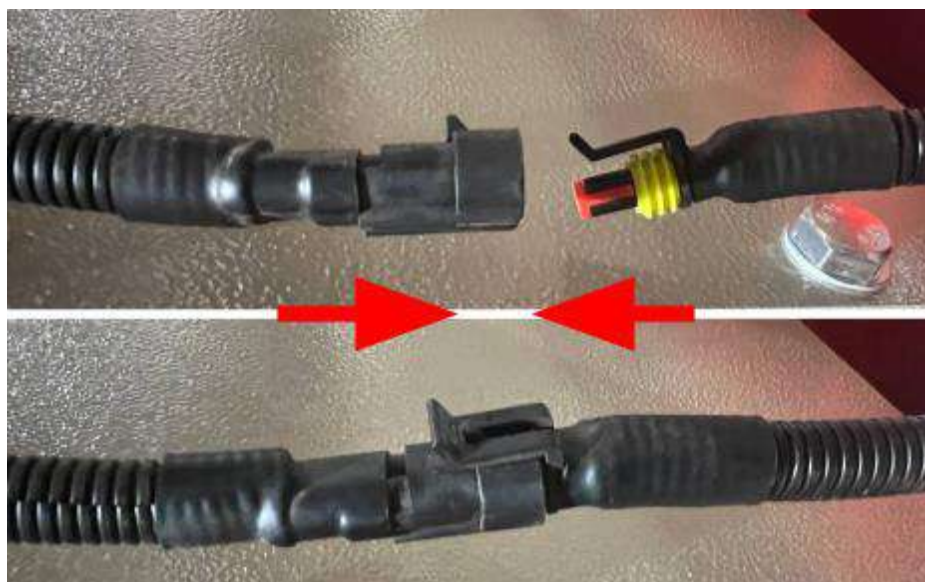
Рисунок 19. Підключення проводки кінцевого вимикача
