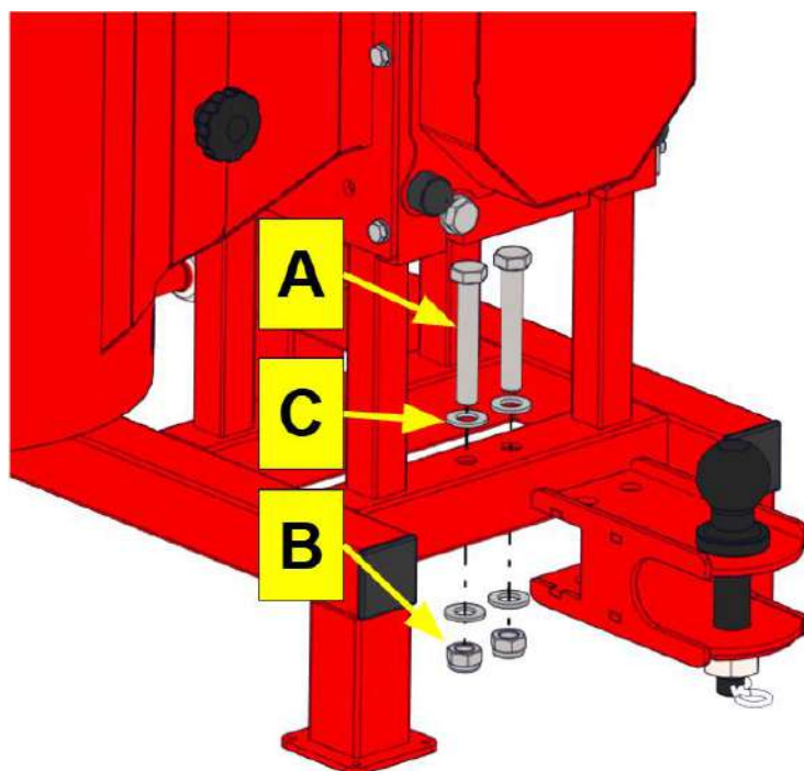
Рисунок 18. Встановлення фаркопа
