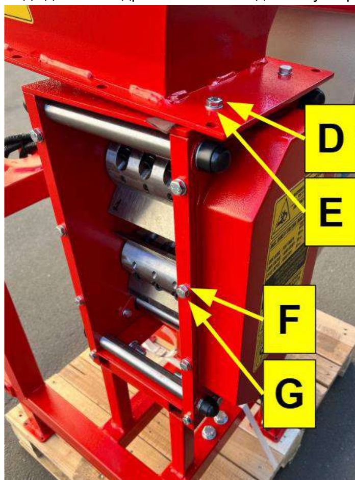
Рисунок 15. Від'єднання вихідного бункера
