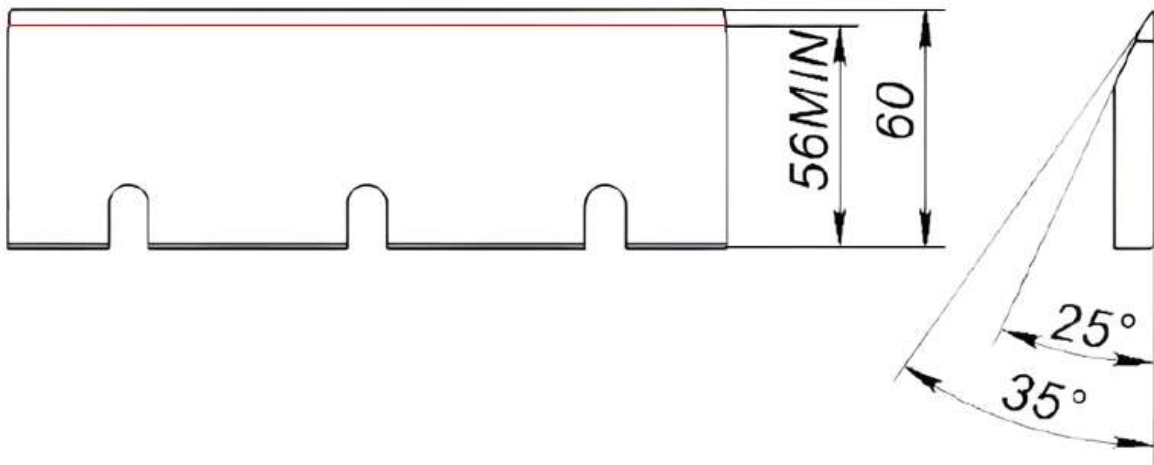
Рисунок 22. Схема заточування ножа
