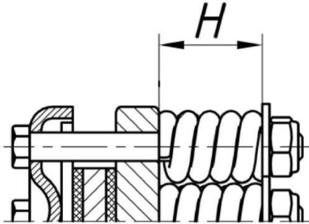
Рисунок 21. Регулювання дискової фрикційної муфти
