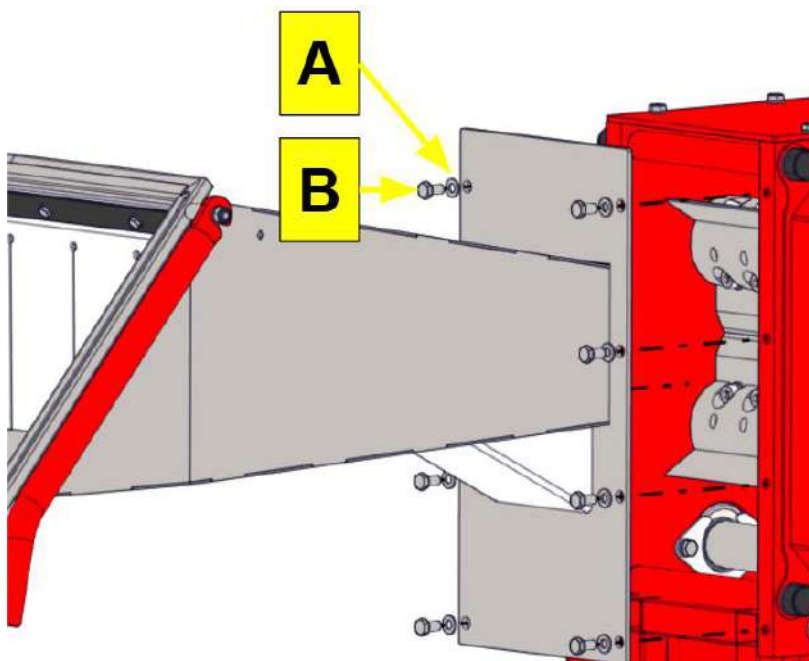
Рисунок 16. Встановлення вхідного бункера
