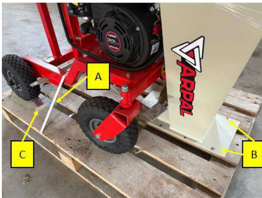
Рисунок 13. Від'єднання подрібнювача та вхідного бункера від палети
