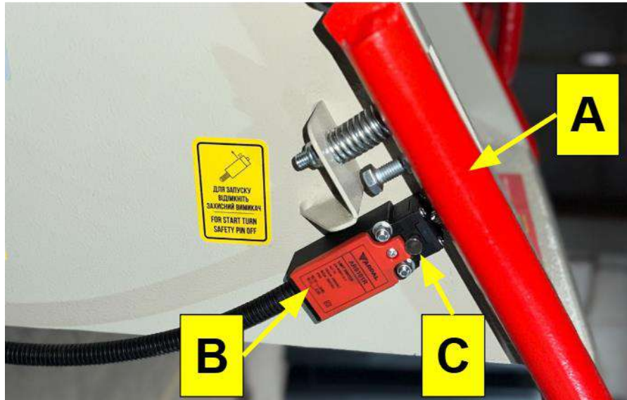
Рисунок 20. Кінцевий вимикач
