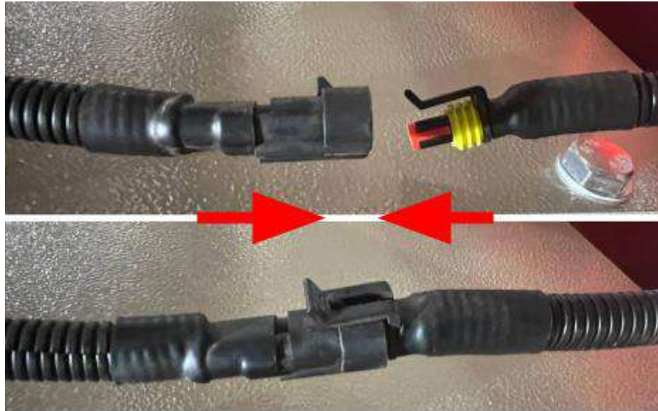
Рисунок 16. Підключення проводки кінцевого вимикача
