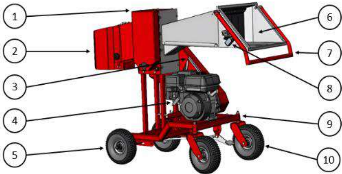
Рисунок 1. Загальний вигляд машини
