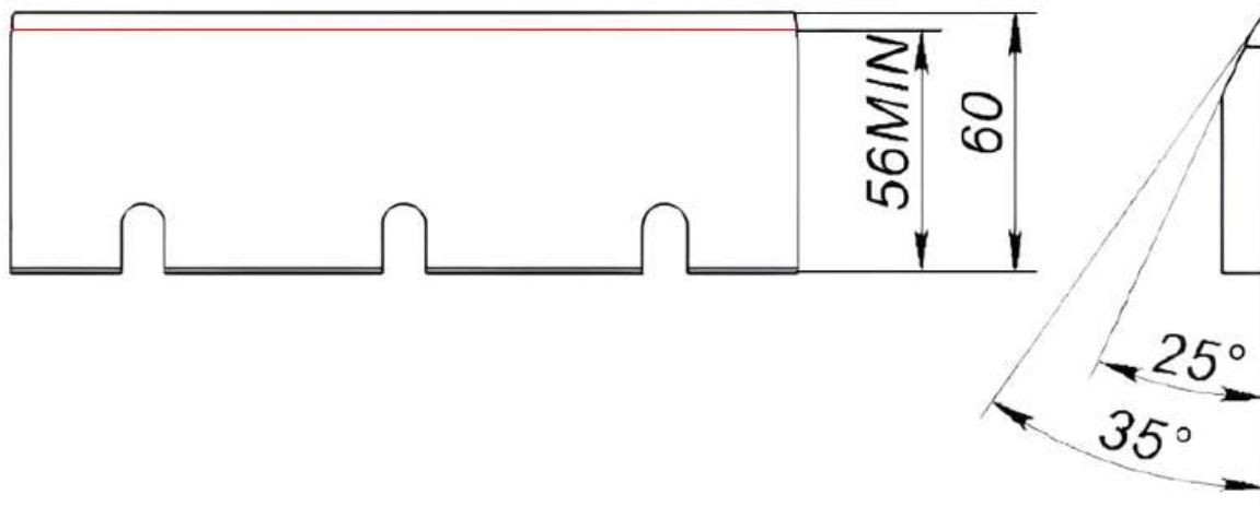
Рисунок 23. Схема заточування ножа
