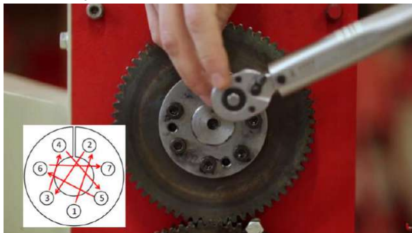
Рисунок 25. Затягування конусної муфти
