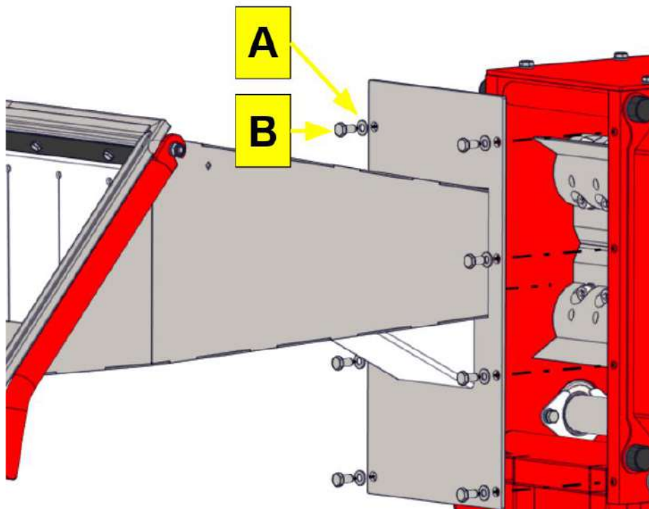
Рисунок 15. Встановлення вхідного бункера
